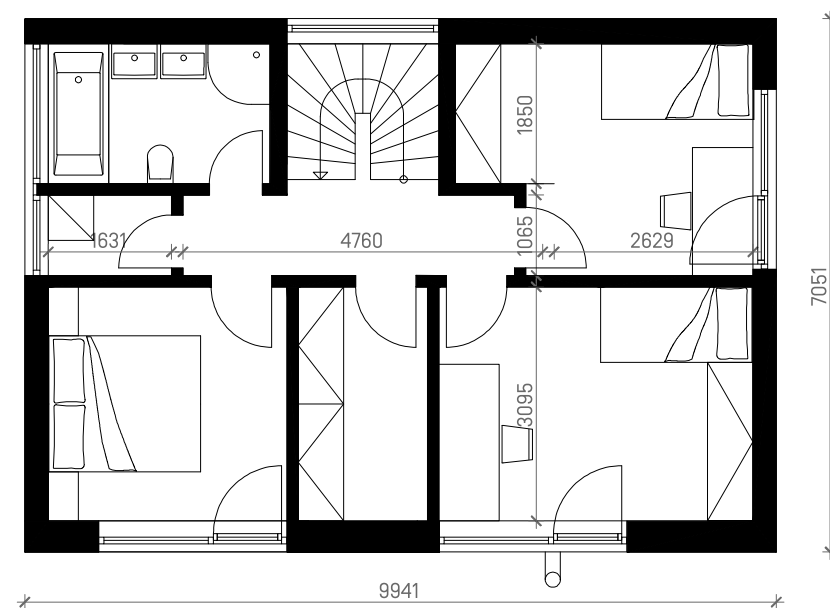
1. PATRO +1 m
