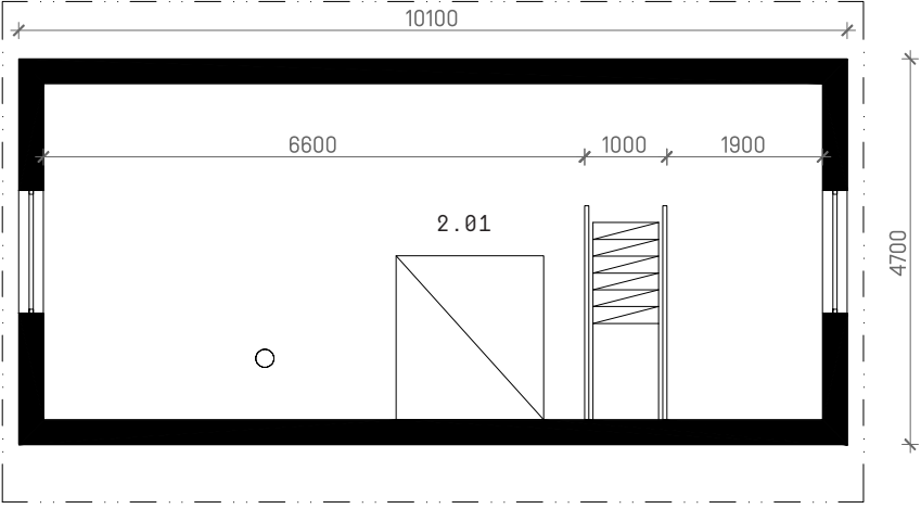
Podkroví M 1:100
