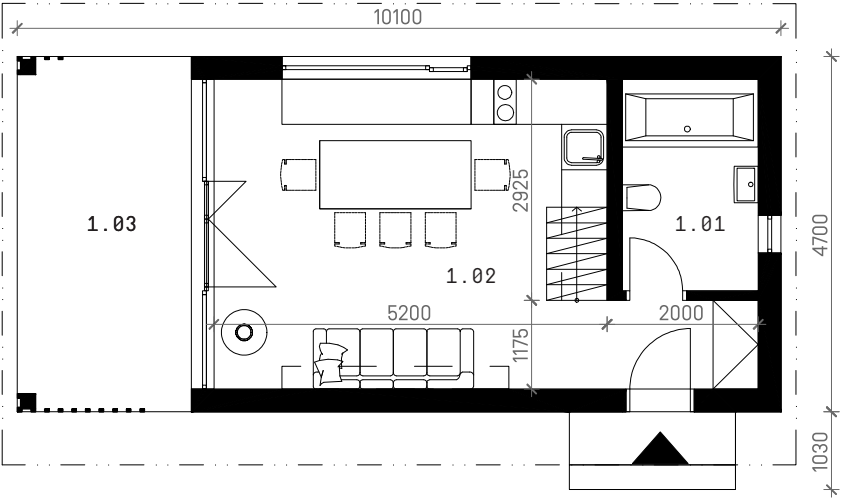
Přízemí M 1:100
